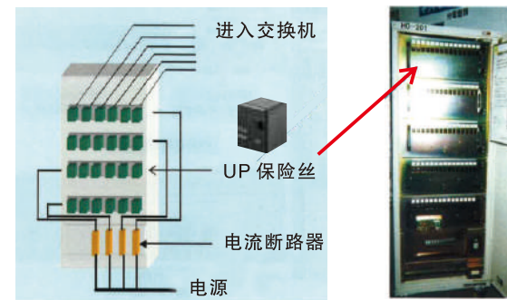
直流配电盘
