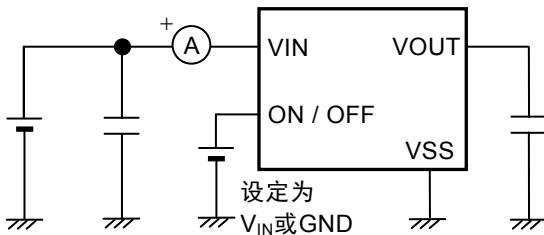
图12 测定电路2
