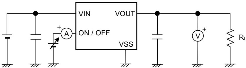
图14 测定电路4
