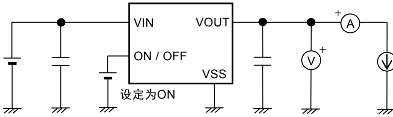
图11 测定电路1
