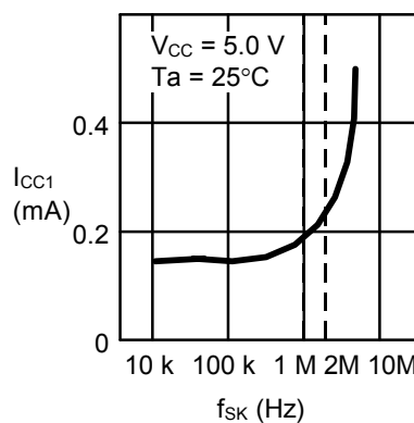
1.6 读出时消耗电流 I_{CC1} —时钟频率 f_{SK}
