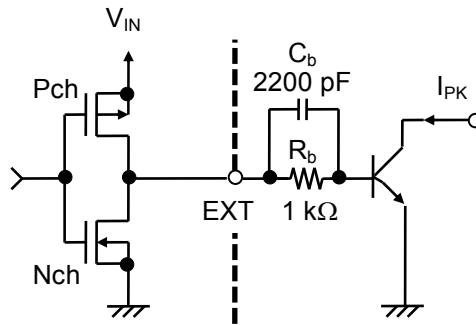
图 11 外接晶体管周围电路
