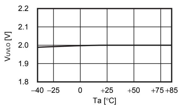
2. 15 V_{UVLO} - T_a
