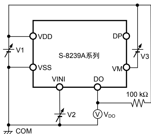
图4 测定电路1
