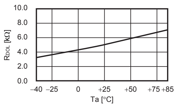
3. 1 R_{DOL} - T_a
