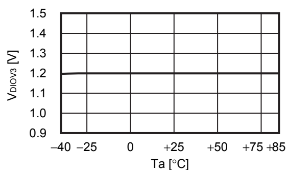
2.3 V_{DIOV3} - T_a
