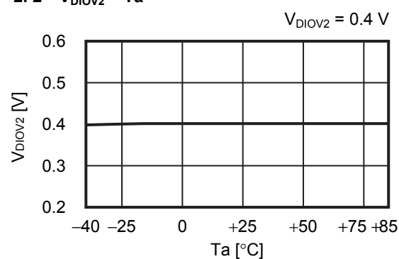
2.2 V_{DIOV2} - T_a
