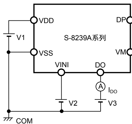
图7 测定电路4
