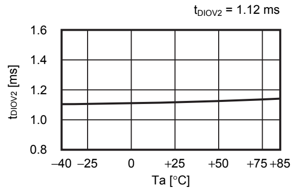
2.10 t_{DIOV2} - T_a
