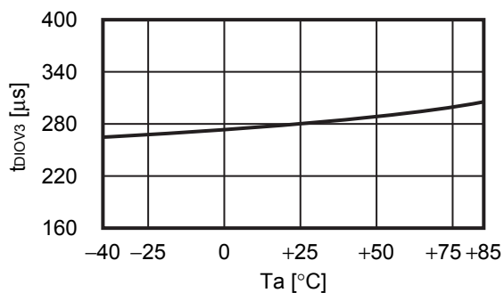
2.11 t_{DIOV3} - T_a
