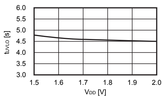
2. 16 t_{UVLO} - V_{DD}
