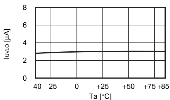
1.3 I_{UVLO} - T_a
