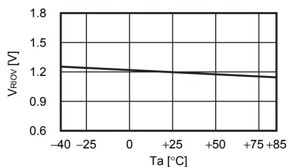
2.4 V_{RIOV} - T_a
