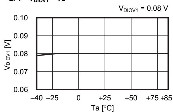
2.1 V_{DIOV1} - T_a
