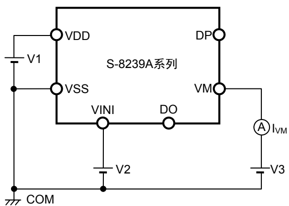
图6 测定电路3
