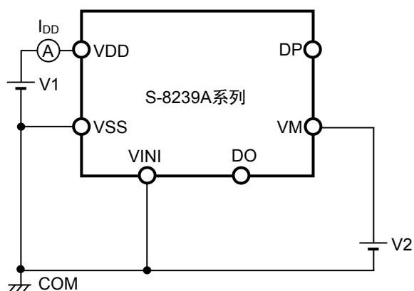
图5 测定电路2
