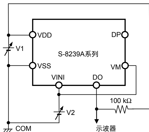
图8 测定电路5
