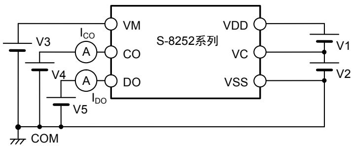
图8 测定电路4
