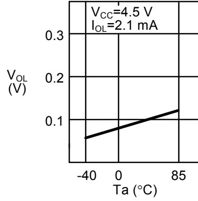
1. 20 低电位输出电压V OL —周围温度Ta
