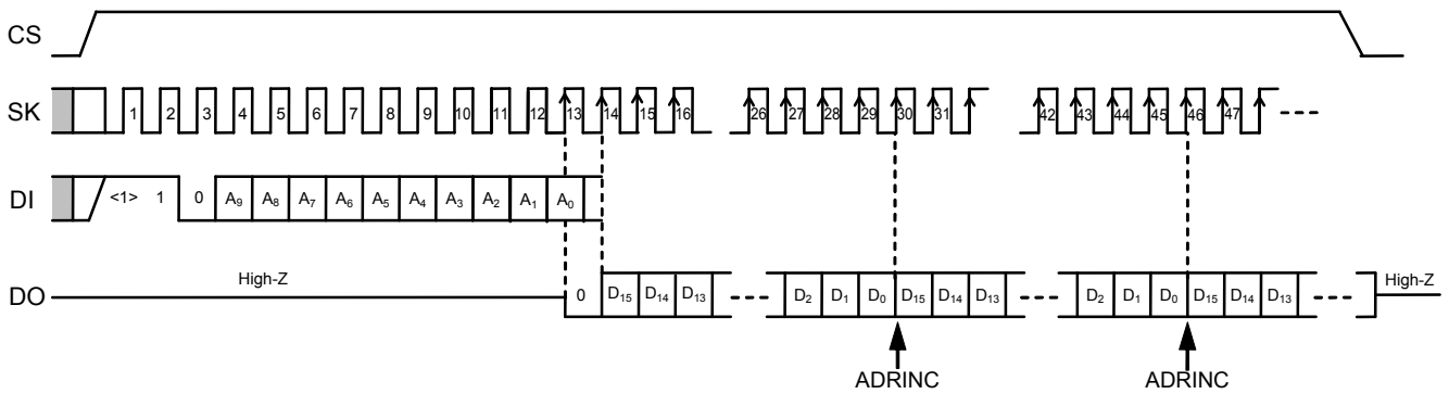
图5 读出定时
