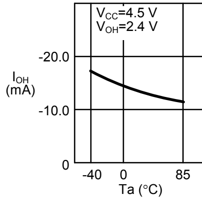
1. 22 高电位输出电流I OH —周围温度Ta
