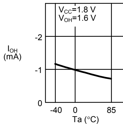
1. 24 高电位输出电流I OH —周围温度Ta
