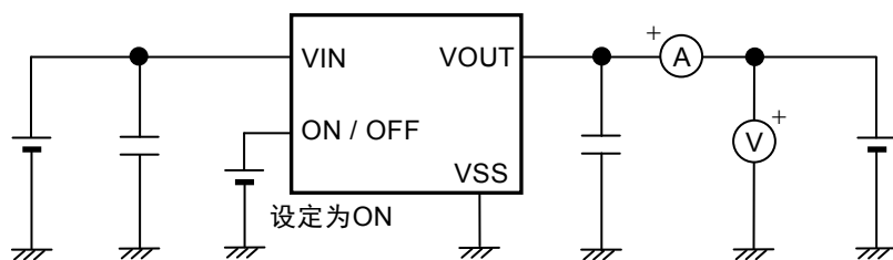
图12 测定电路3
