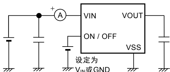
图11 测定电路2
