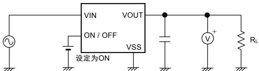
图14 测定电路5
