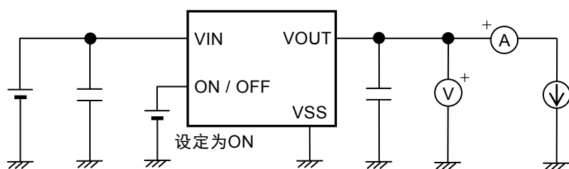
图10 测定电路1
