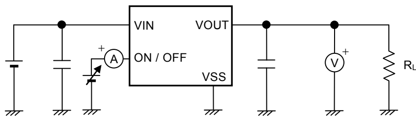
图13 测定电路4
