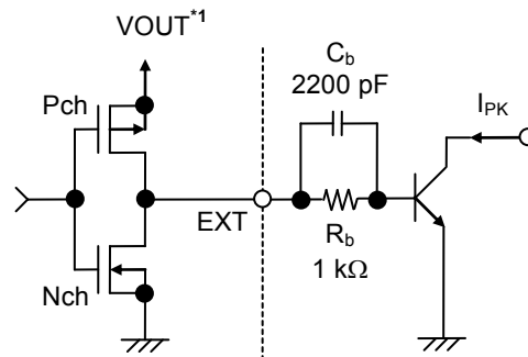
图 18 外接晶体管外围电路
