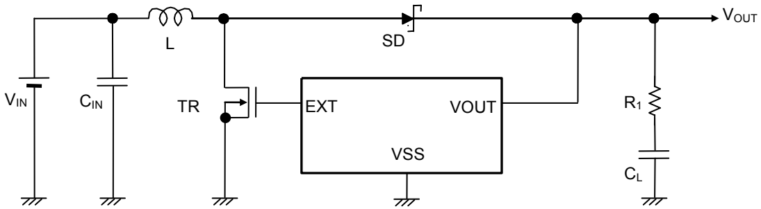
图26 陶瓷电容器使用电路示例
