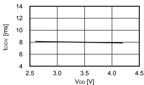
2. 11 t_{CLOV} - V_{DD}
