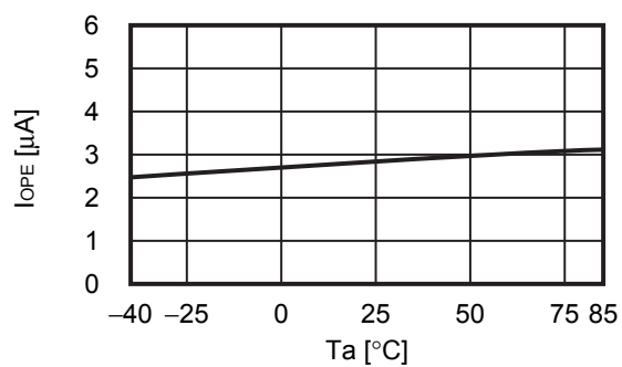
1.1 I_{OPE} - T_a
