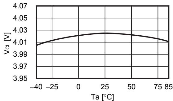
2.2 V_{CL} - T_a
