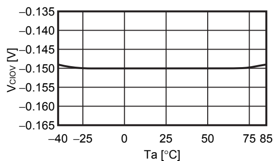
2. 10 V_{CLOV} - T_a
