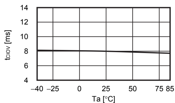
2. 12 t_{CLOV} - T_a
