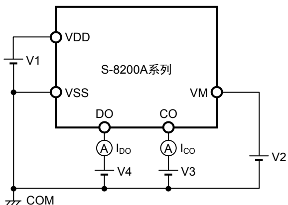
图8 测定电路4
