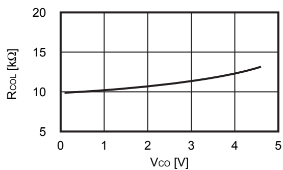
3.2 R_{COL} - V_{CO}
