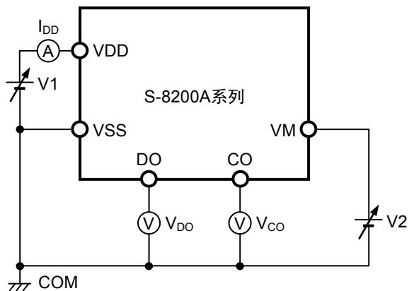
图6 测定电路2
