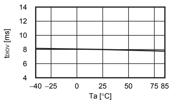
2. 9 t_{BIOV} - T_a
