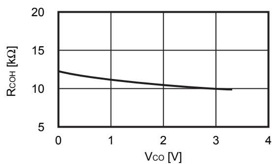
3.1 R_{COH} - V_{CO}
