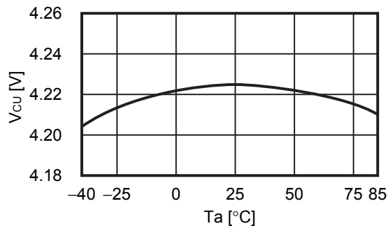
2.1 V_{CU} - T_a
