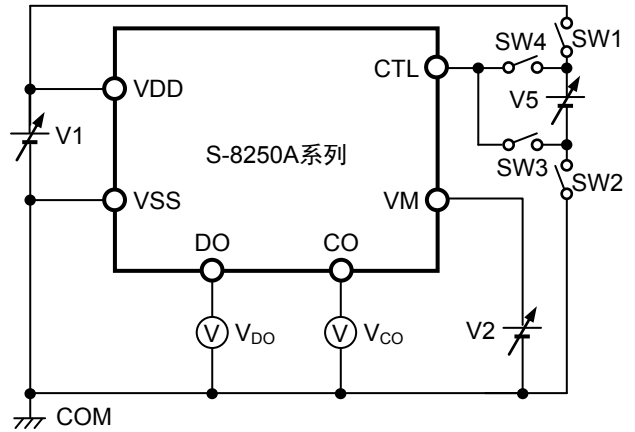
图5 测定电路2
