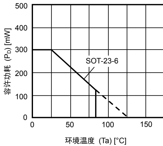
图11 封装容许功耗
