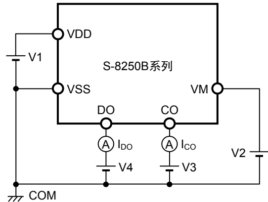
图7 测定电路4
