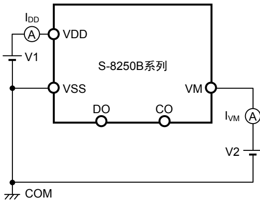
图6 测定电路3
