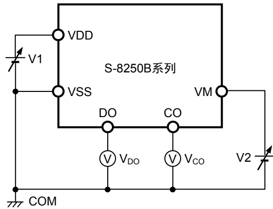
图5 测定电路2
