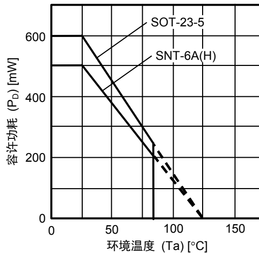
图5 封装容许功耗 (基板安装时)
