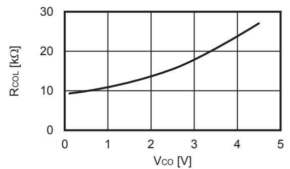
4.2 R_{COL} - V_{CO}
