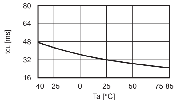
3.2 t_{CL} - T_a
