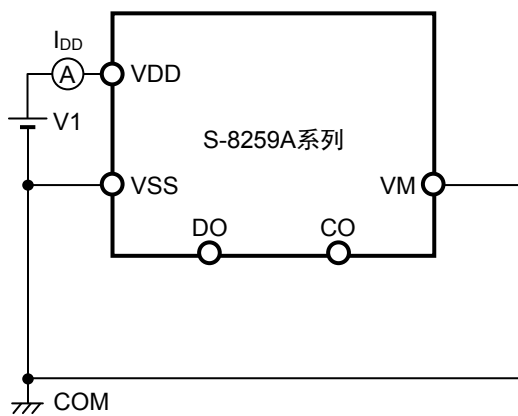
图6 测定电路3
