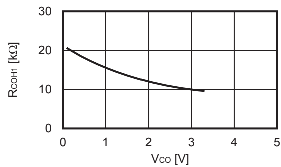
4.1 R_{COH1} - V_{CO}
