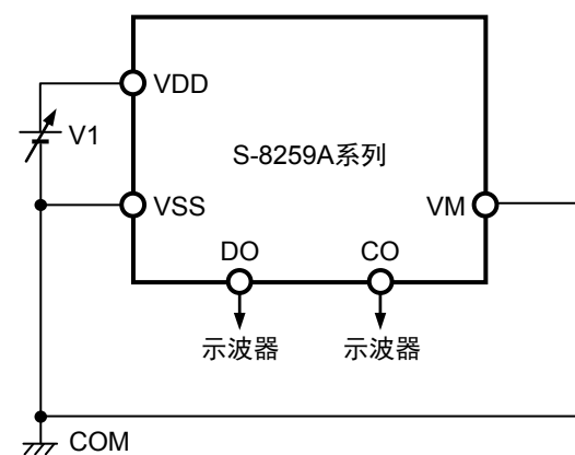
图8 测定电路5
