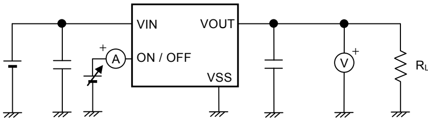
图12 测定电路4
