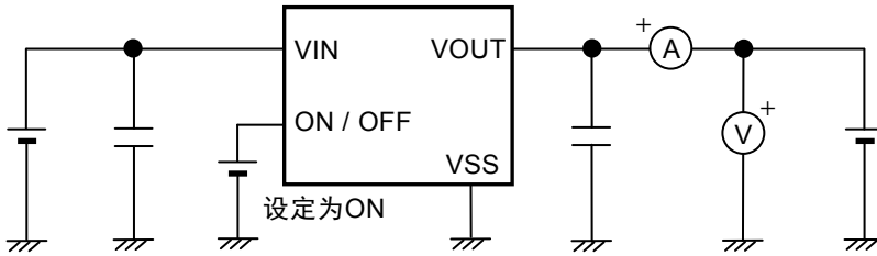
图11 测定电路3
