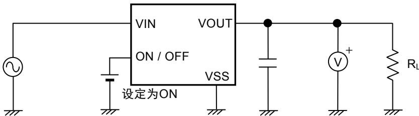
图13 测定电路5
