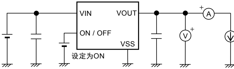
图9 测定电路1
