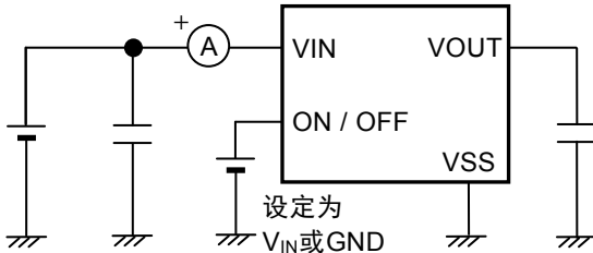
图10 测定电路2
