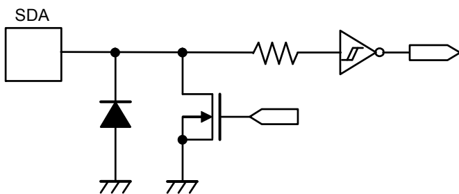
图5 SDA端子
