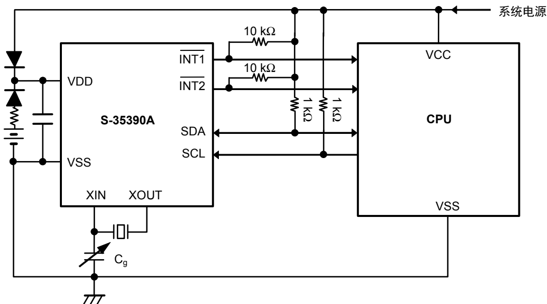
图49 应用电路2
