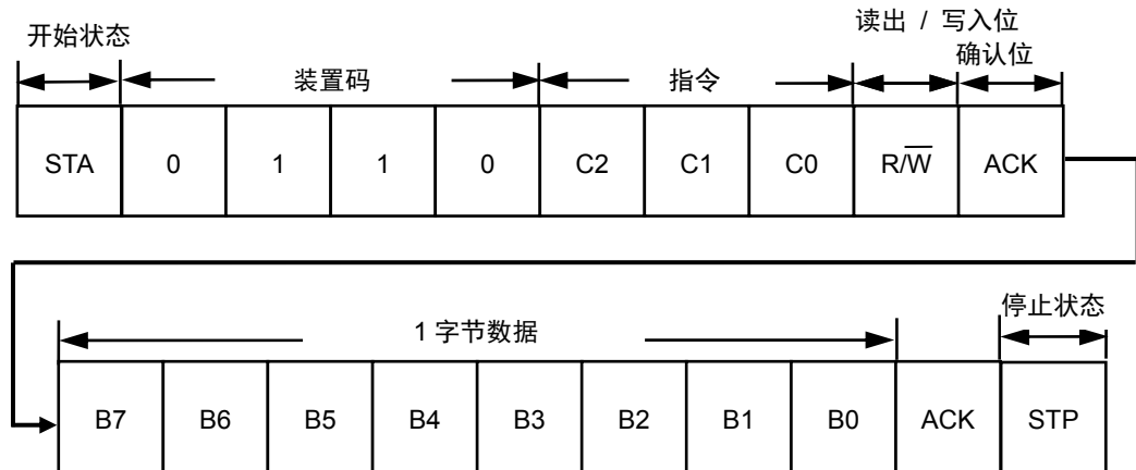
图10 通信数据
