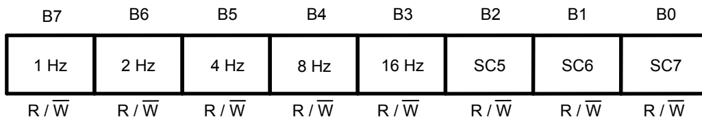
图15 INT1寄存器 (频率设定数据)
