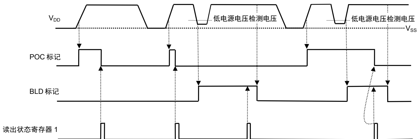
图24 POC标记和BLD标记
