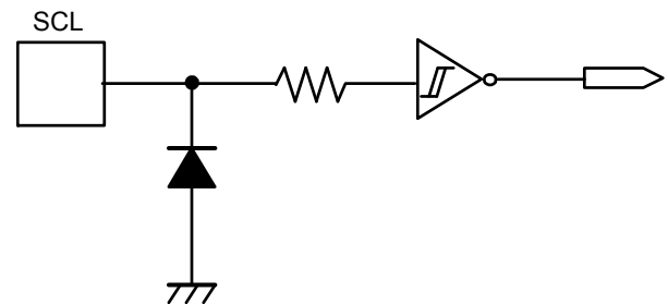
图6 SCL端子
