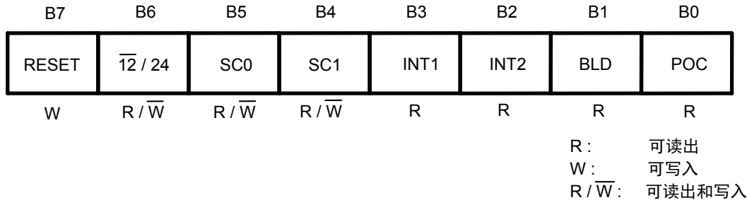
图12 状态寄存器1
