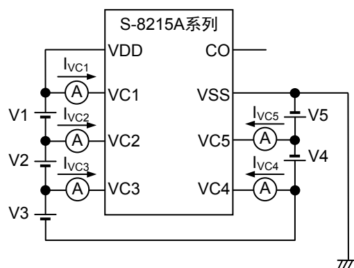
图8 测定电路4
