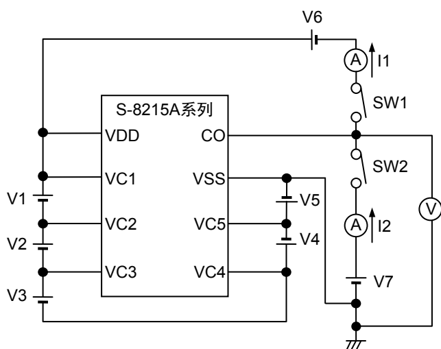
图9 测定电路5
