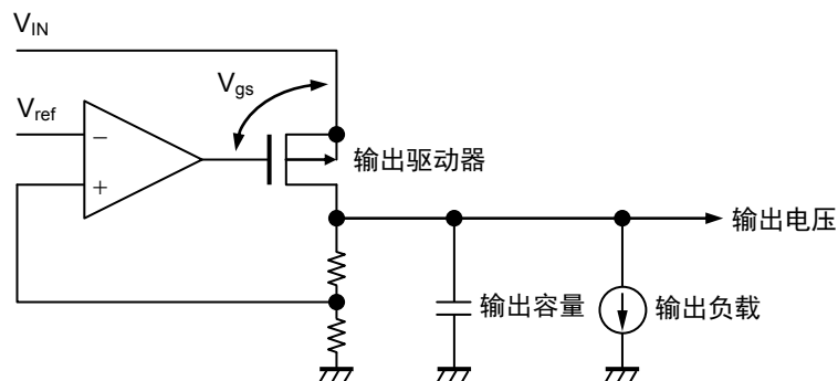
图13 电路图
