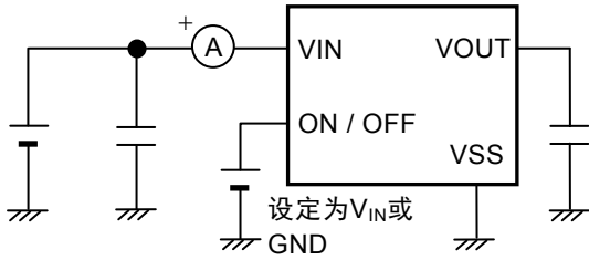
图6 测定电路2
