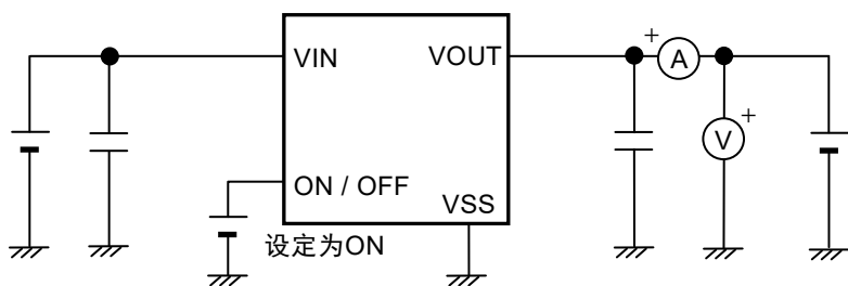
图7 测定电路3
