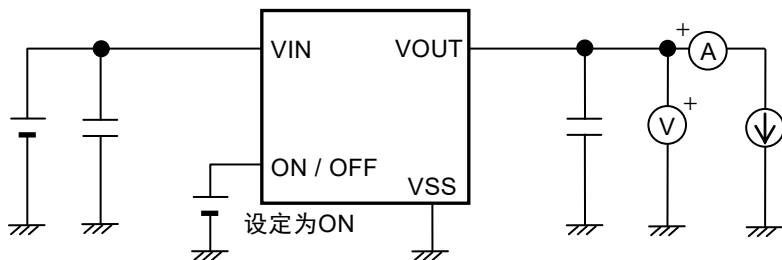
图5 测定电路1
