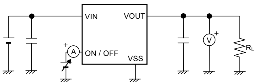
图8 测定电路4
