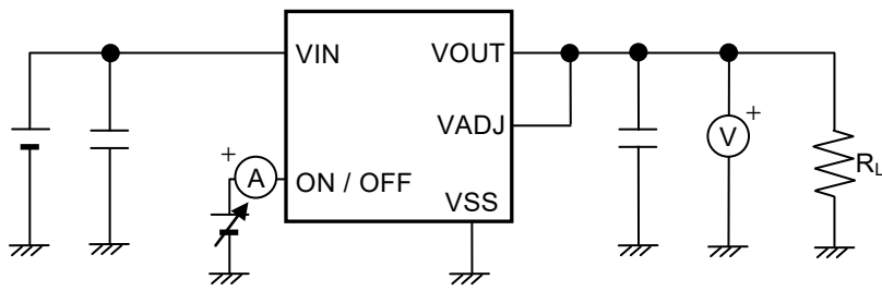
图14 测定电路10
