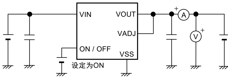
图13 测定电路9
