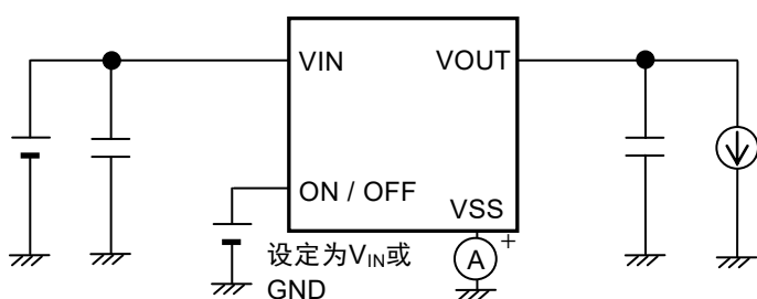
图6 测定电路2
