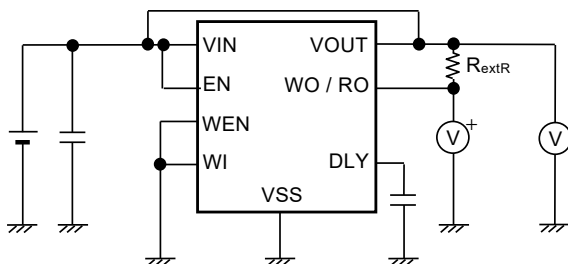
图13 测定电路5
