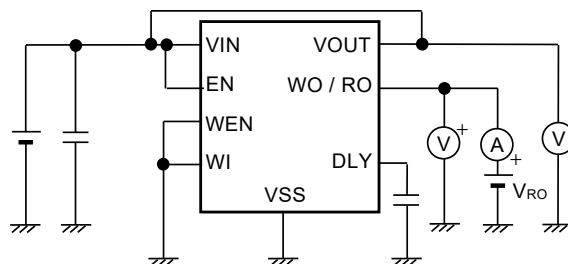
图14 测定电路6
