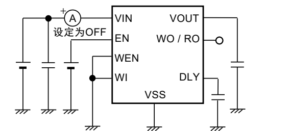
图18 测定电路10
