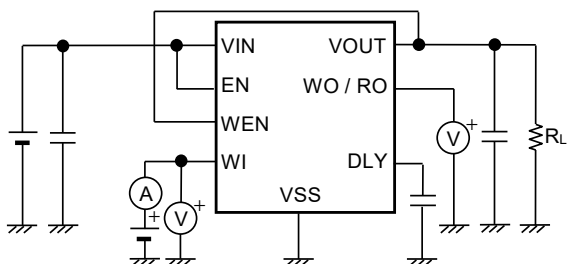
图15 测定电路7
