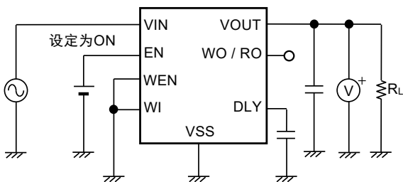
图11 测定电路3
