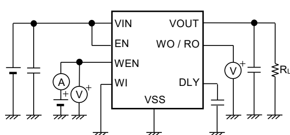
图16 测定电路8
