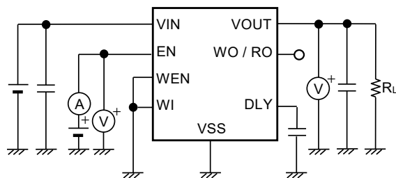
图12 测定电路4
