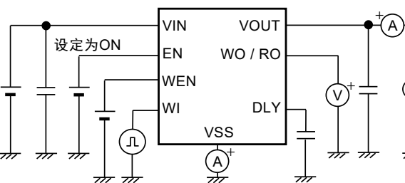
图17 测定电路9
