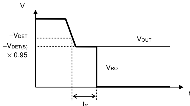
图7 复位反应时间
