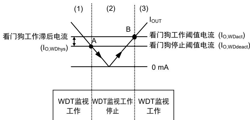
图41 自律看门狗工作功能
