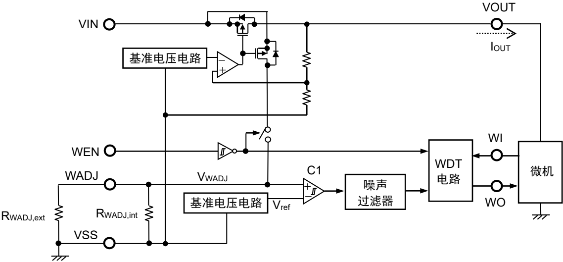
图40 输出电流检测电路工作说明图
