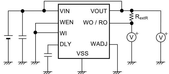
图15 测定电路4
