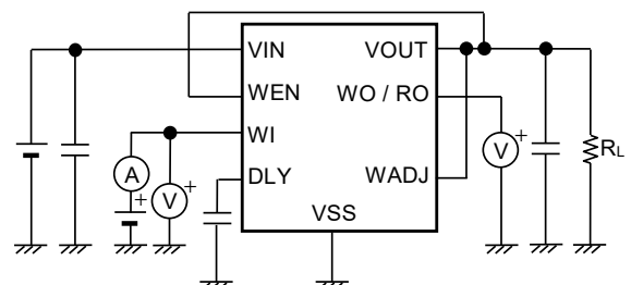
图19 测定电路8
