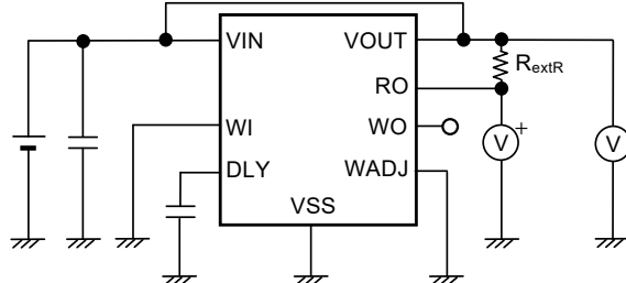
图25 测定电路4
