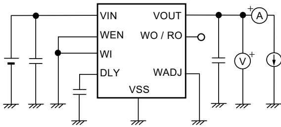
图12 测定电路1
