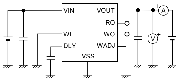
图23 测定电路2
