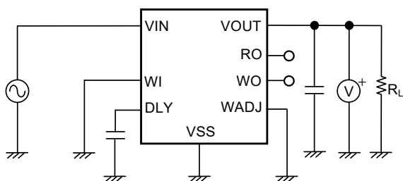
图24 测定电路3
