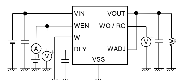
图20 测定电路9
