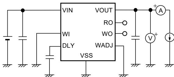
图22 测定电路1
