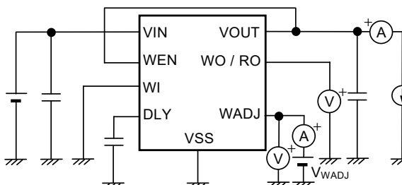
图18 测定电路7
