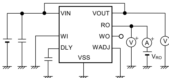
图26 测定电路5
