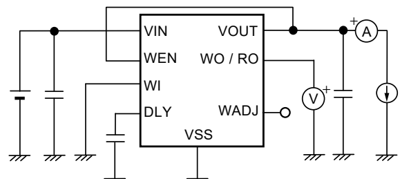
图17 测定电路6
