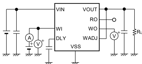
图29 测定电路8
