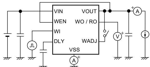
图21 测定电路10
