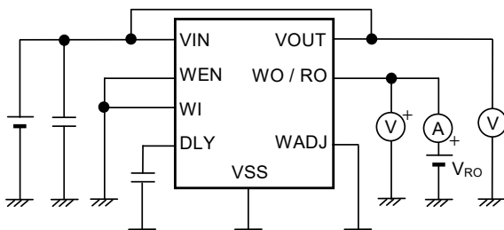
图16 测定电路5
