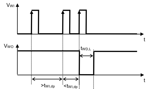
图11 看门狗双脉冲检测时间
