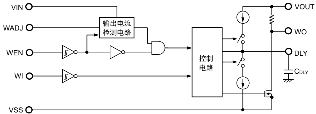
图39 看门狗定时器部分的工作说明图
