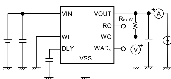
图27 测定电路6
