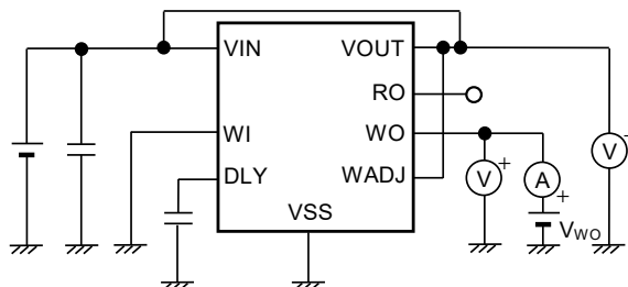
图30 测定电路9
