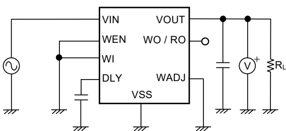
图14 测定电路3
