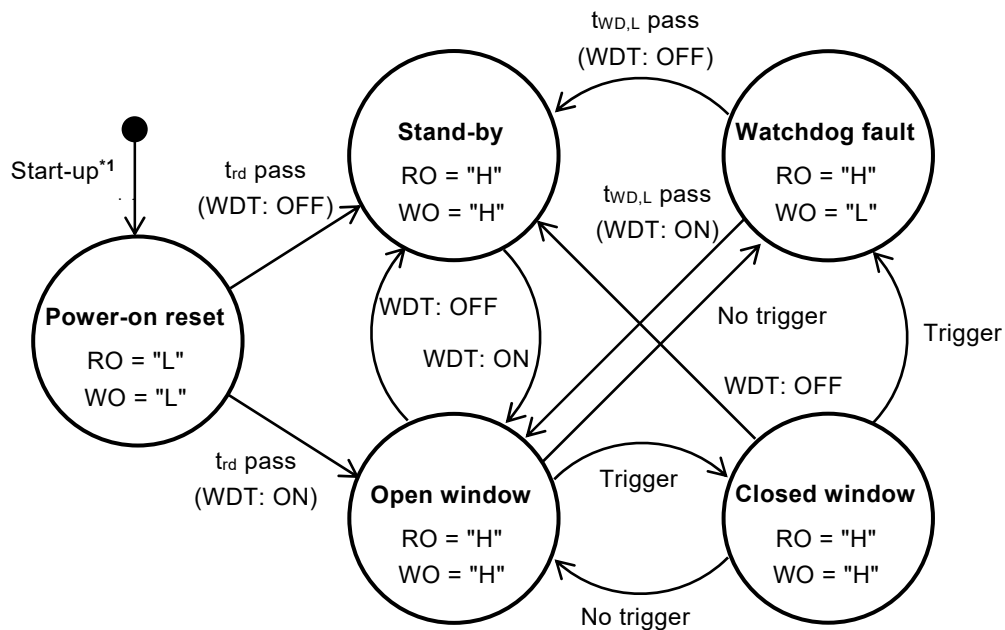
图38 看门狗定时器部分的状态迁移图
