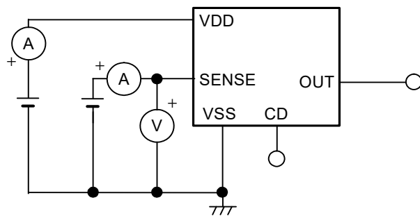
图9 测定电路4
