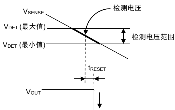
图11 检测电压
