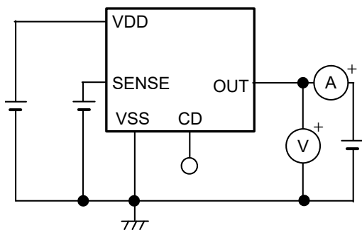
图7 测定电路2
