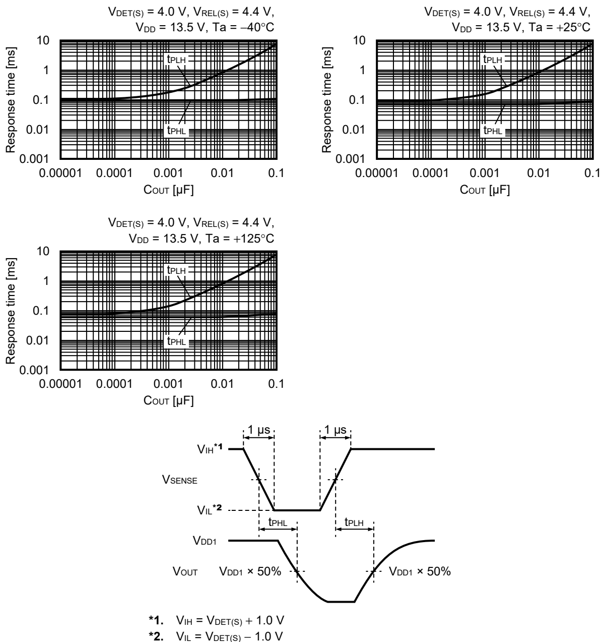
图24 响应时间的测定条件
