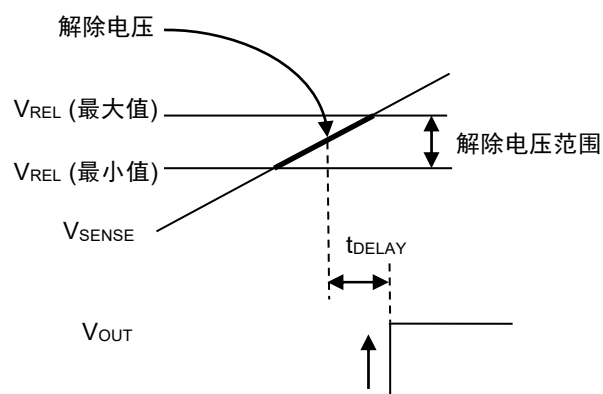
图12 解除电压
