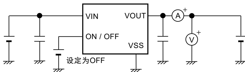
图12 测定电路6
