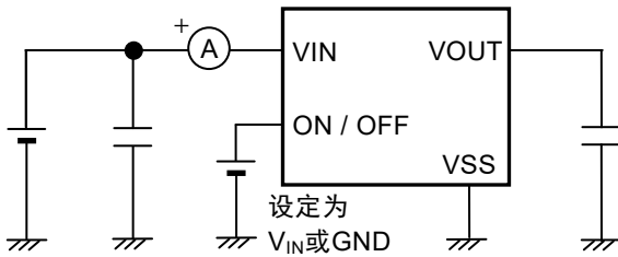
图8 测定电路2
