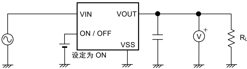
图11 测定电路5
