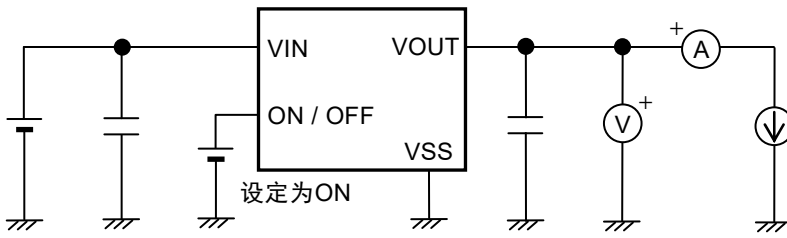
图7 测定电路1
