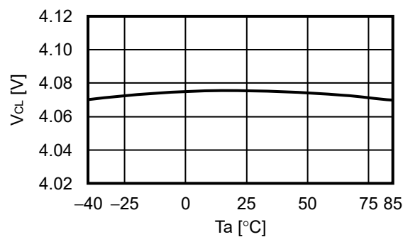
2.2 V_{CL} - T_a
