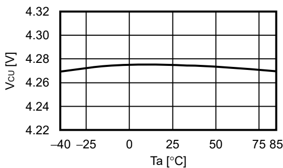
2.1 V_{CU} - T_a
