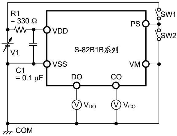
图4 测定电路1
