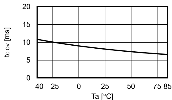
3.10 t_{CI0V} - T_a
