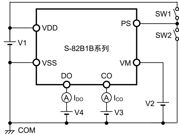
图7 测定电路4
