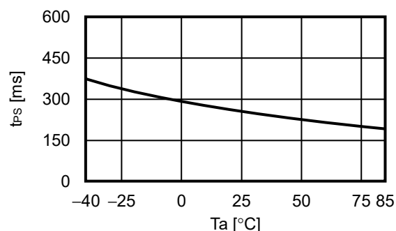
3.12 t_{PS} - T_a
